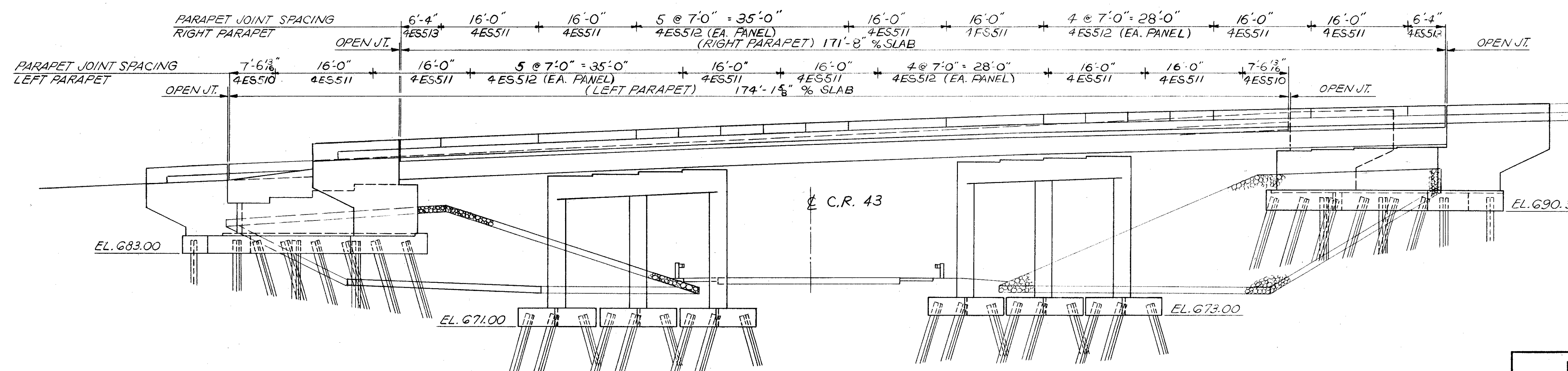
ELEVATION
