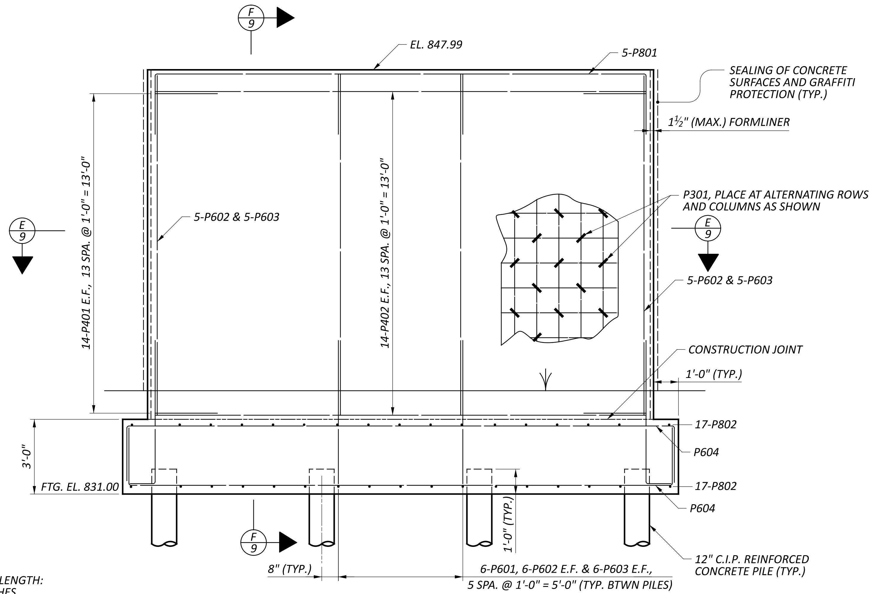
ELEVATION
