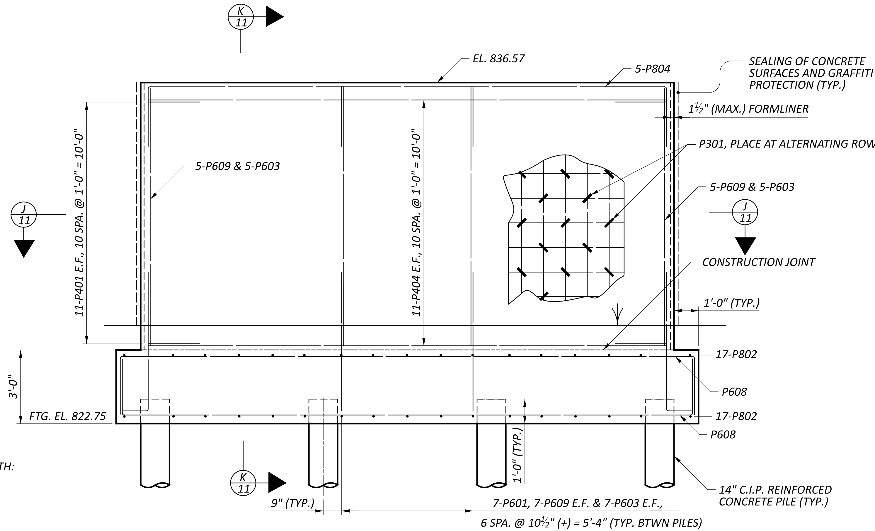
ELEVATION
