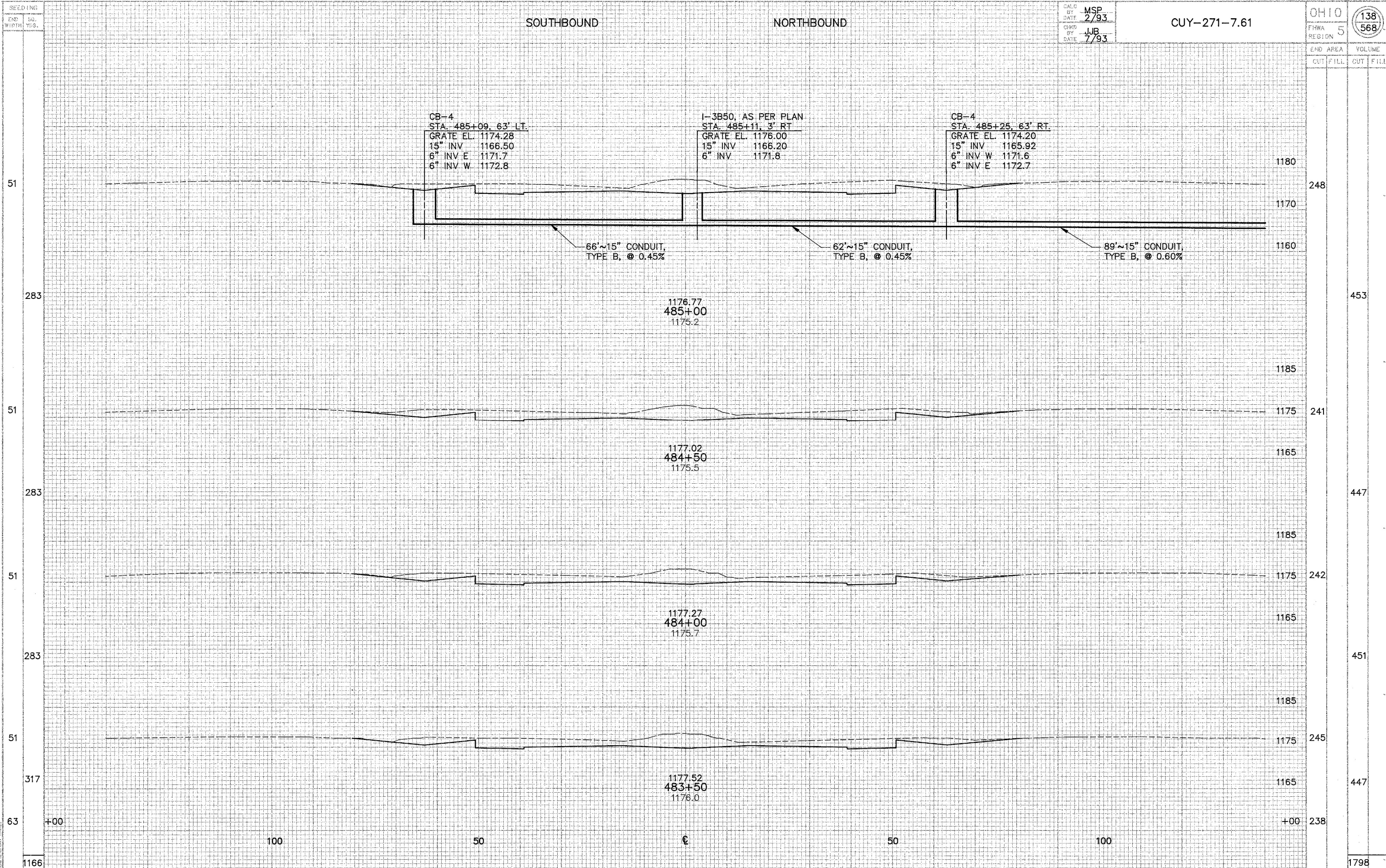
CROSS SECTIONS STA. 483+50 TO STA. 485+00
