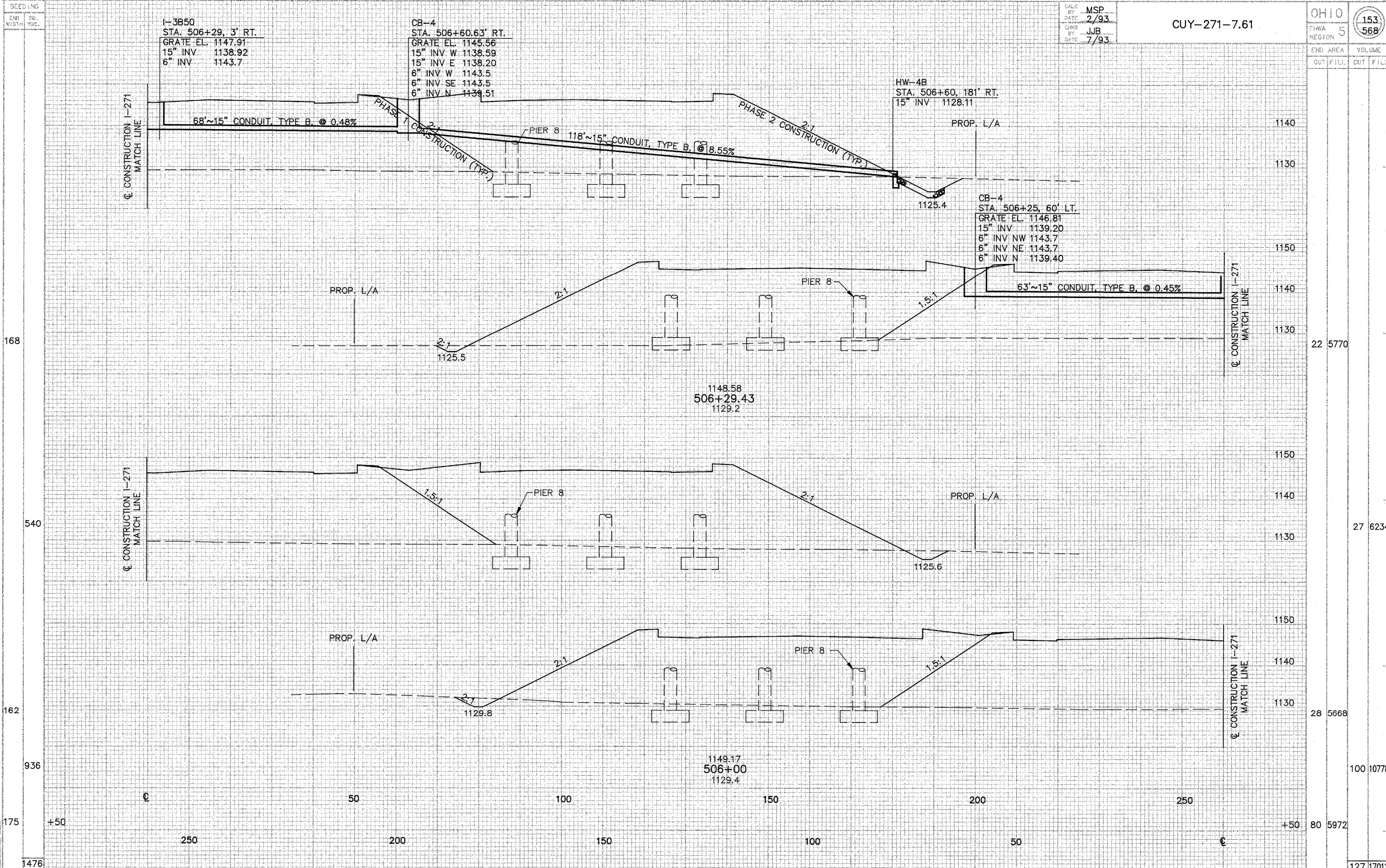
CROSS SECTIONS STA. 506+00 TO STA. 506+29.43
