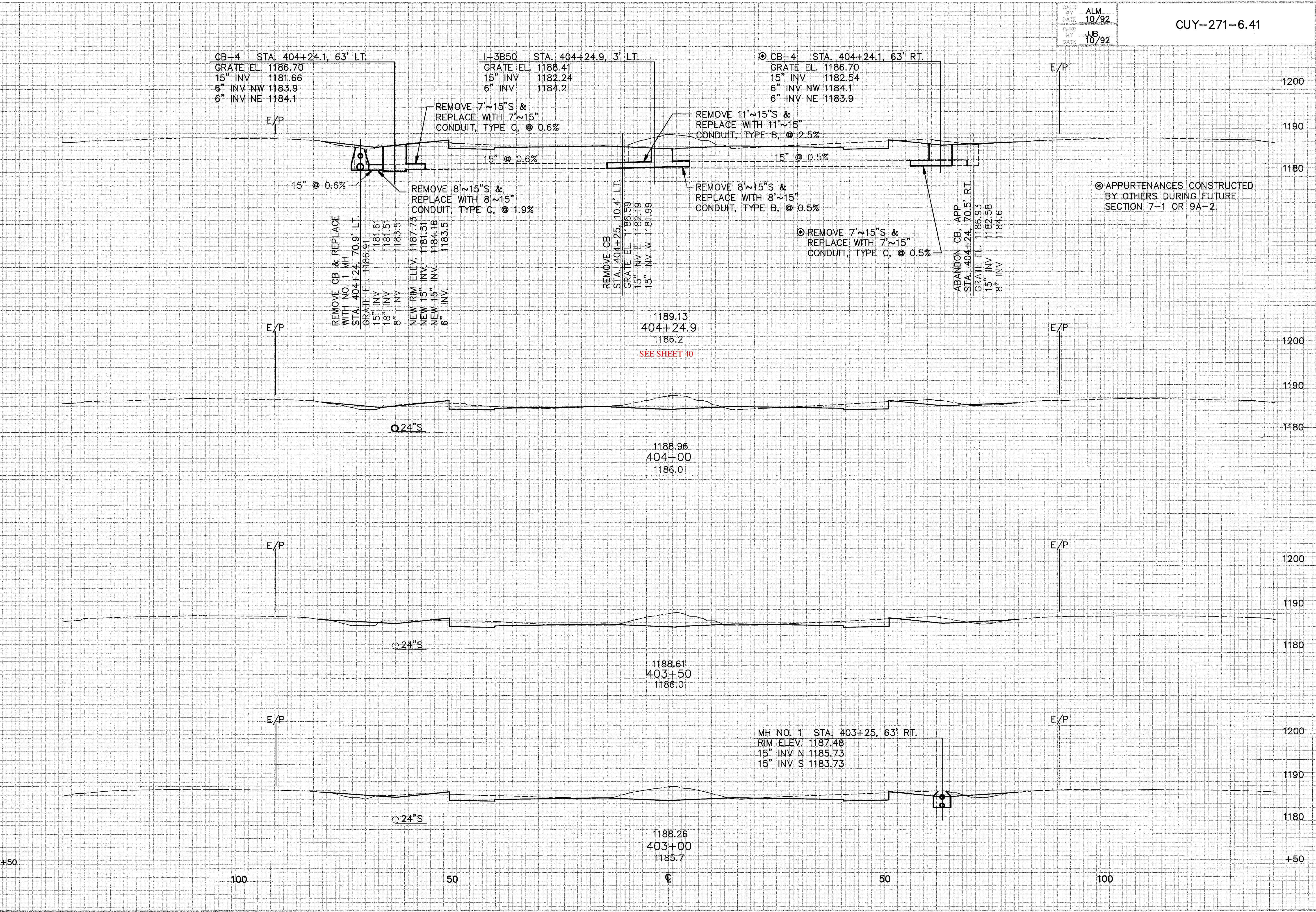
CROSS SECTIONS STA. 403+00 TO STA. 404+24.90
