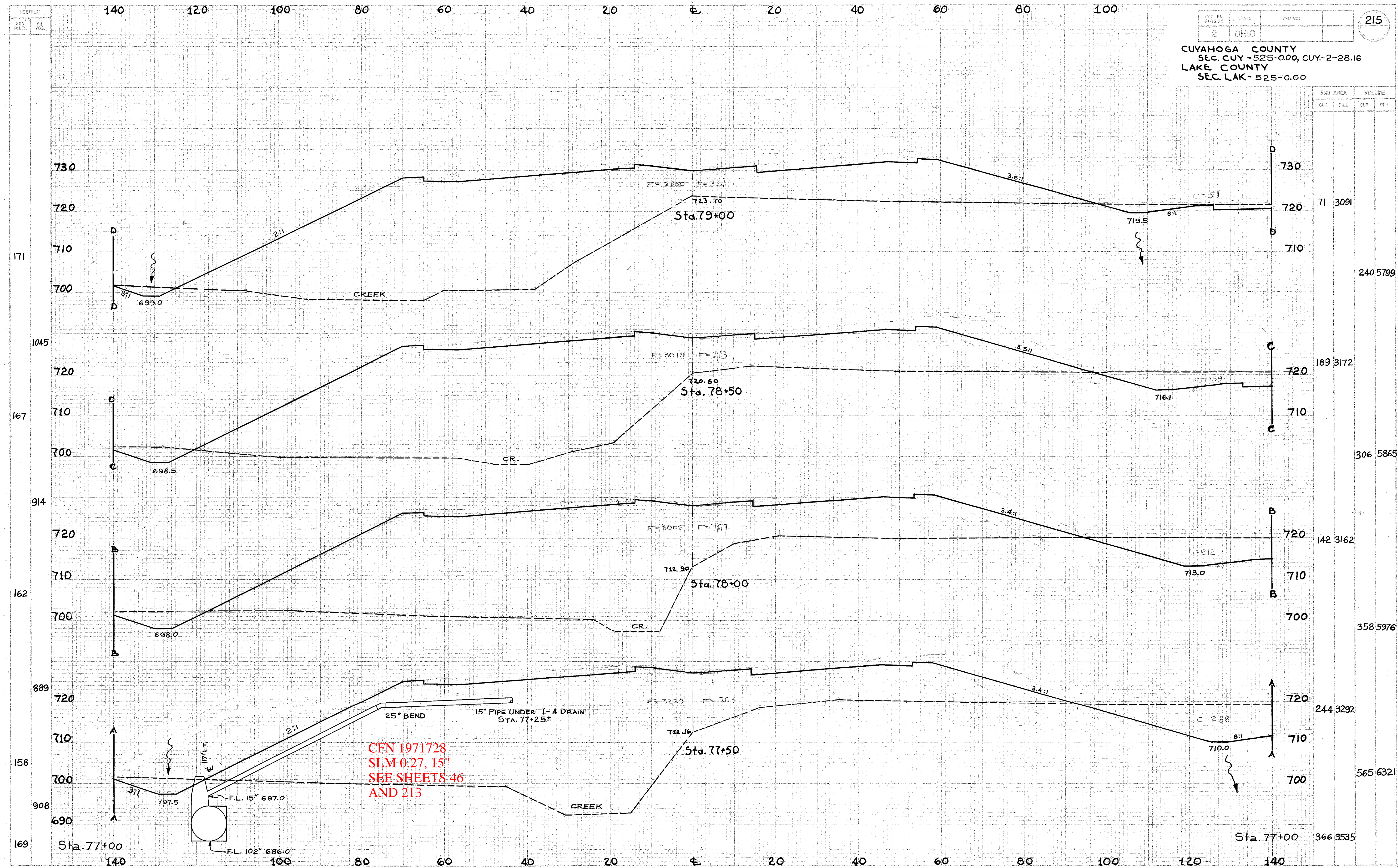
EUCLID SPUR X-SECTIONS STA. 77+50 TO STA. 79+00
