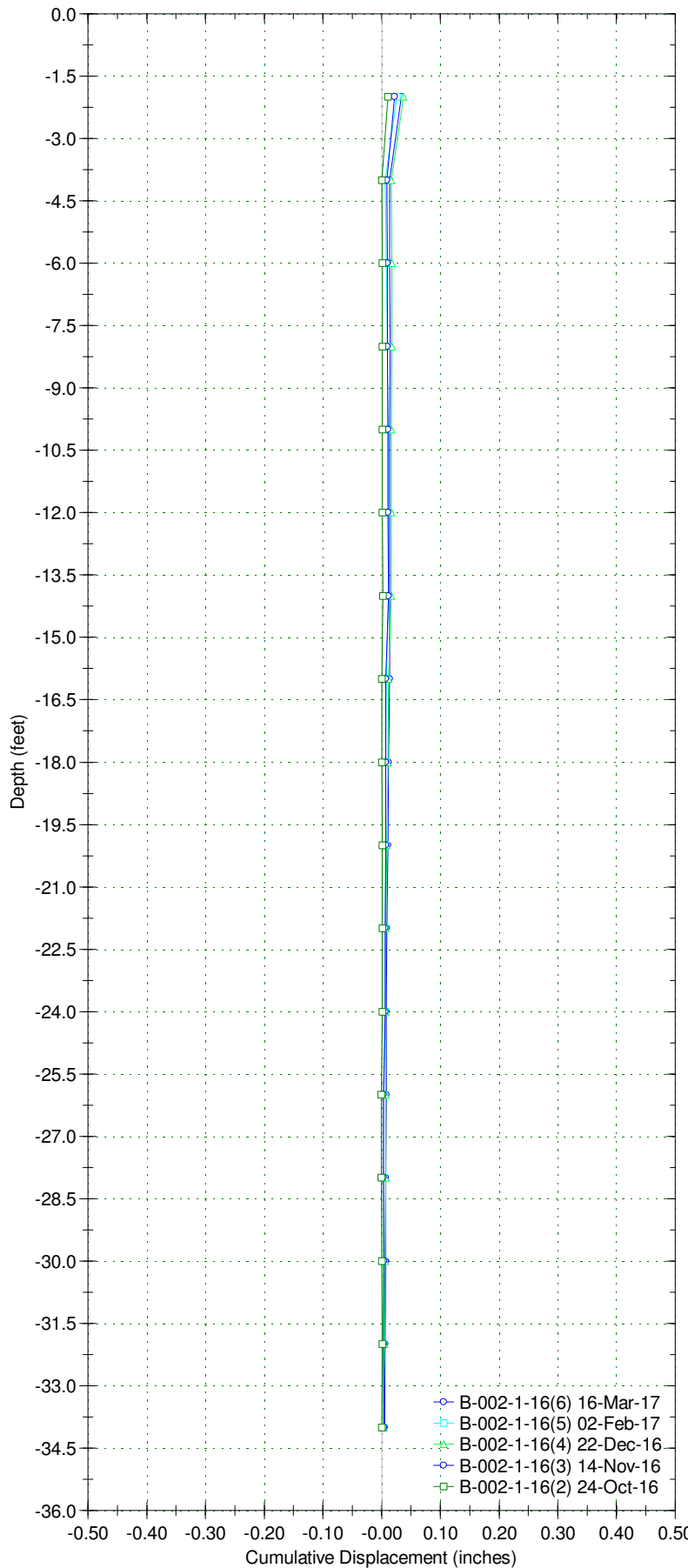
Axis - B
