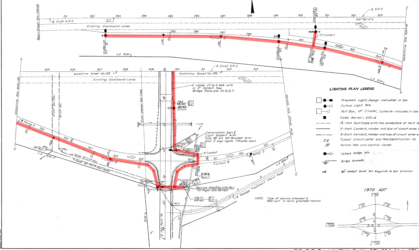
E.B. S.R. 2 - LIGHTING PLAN - STA. 290+00 to STA. 314+00
