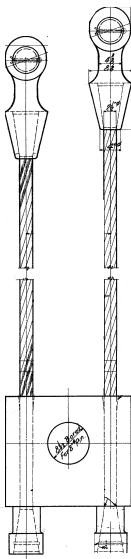
Elevation
