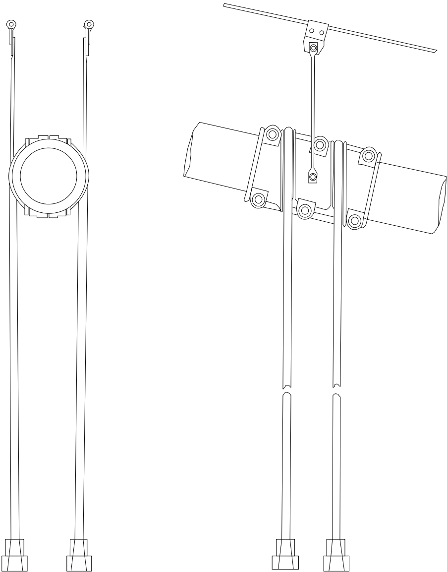
End Elevation
