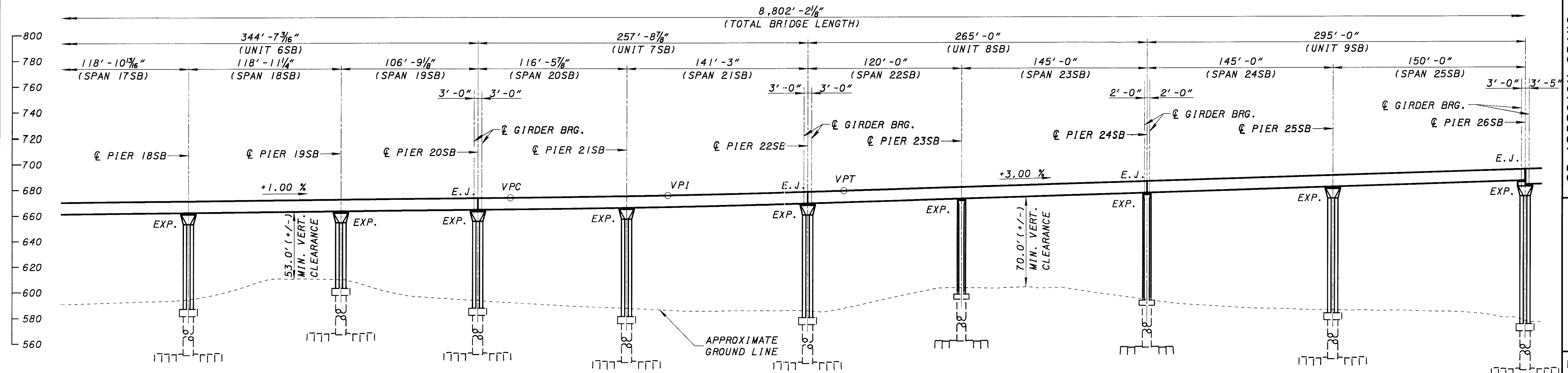
ELEVATION
