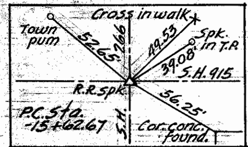
ORIGINAL PLAT
