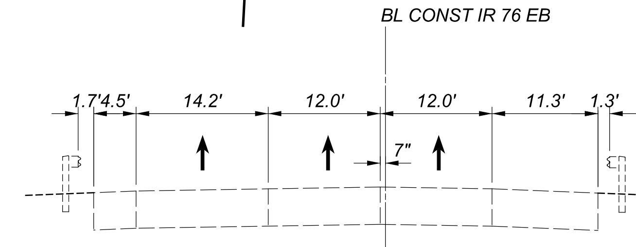
EXISTING SECTION IR 76 SECTION AF-AF STA. 535+00
