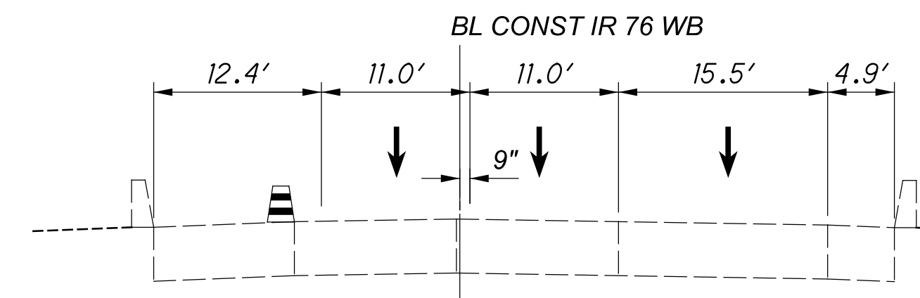
PHASE 3A SECTION AG-AG STA. 539+00
