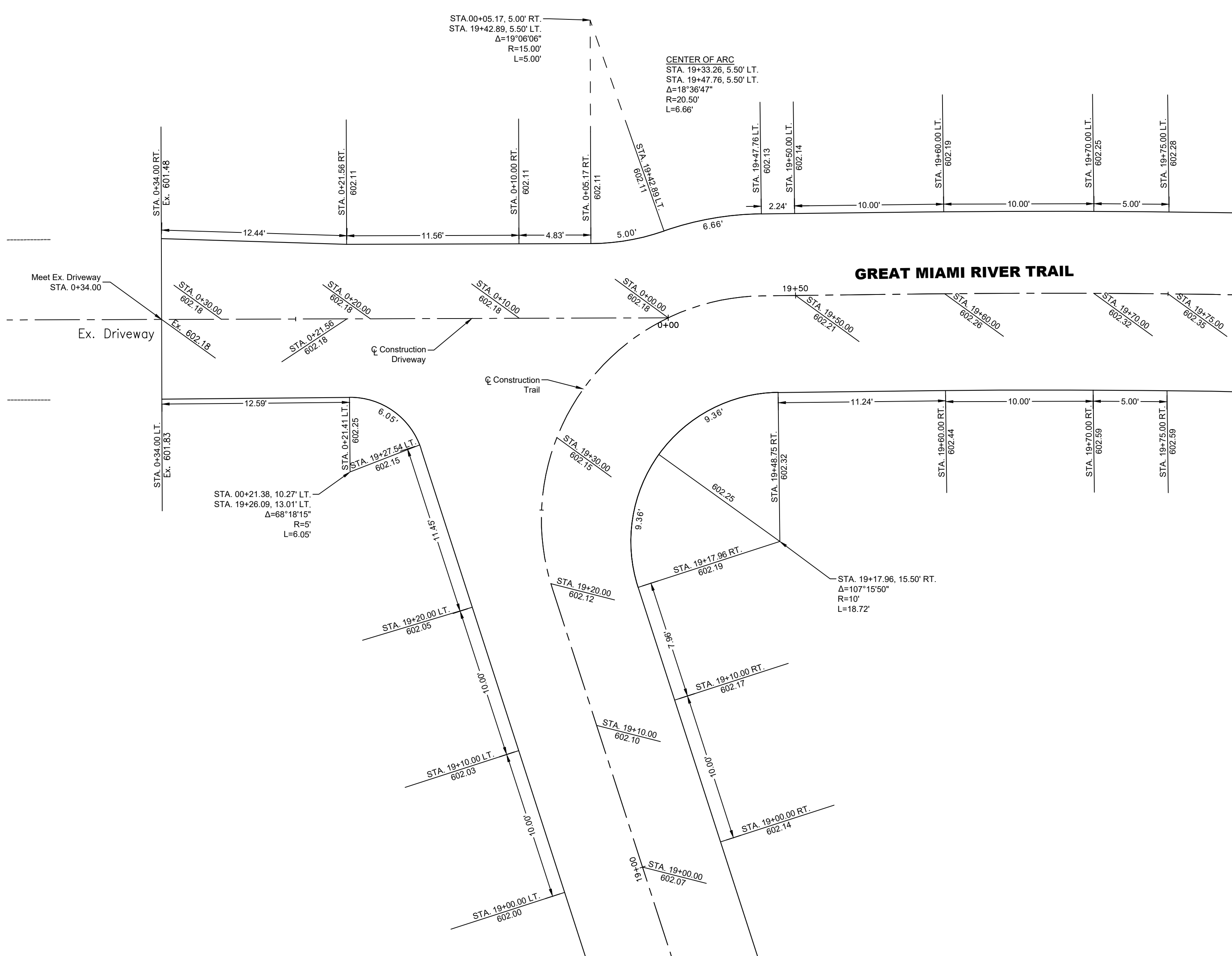
INTERSECTION DETAIL STA. 19+17.96 TO STA. 19+48.07 STA. 0+00.00 TO STA. 0+34.00
