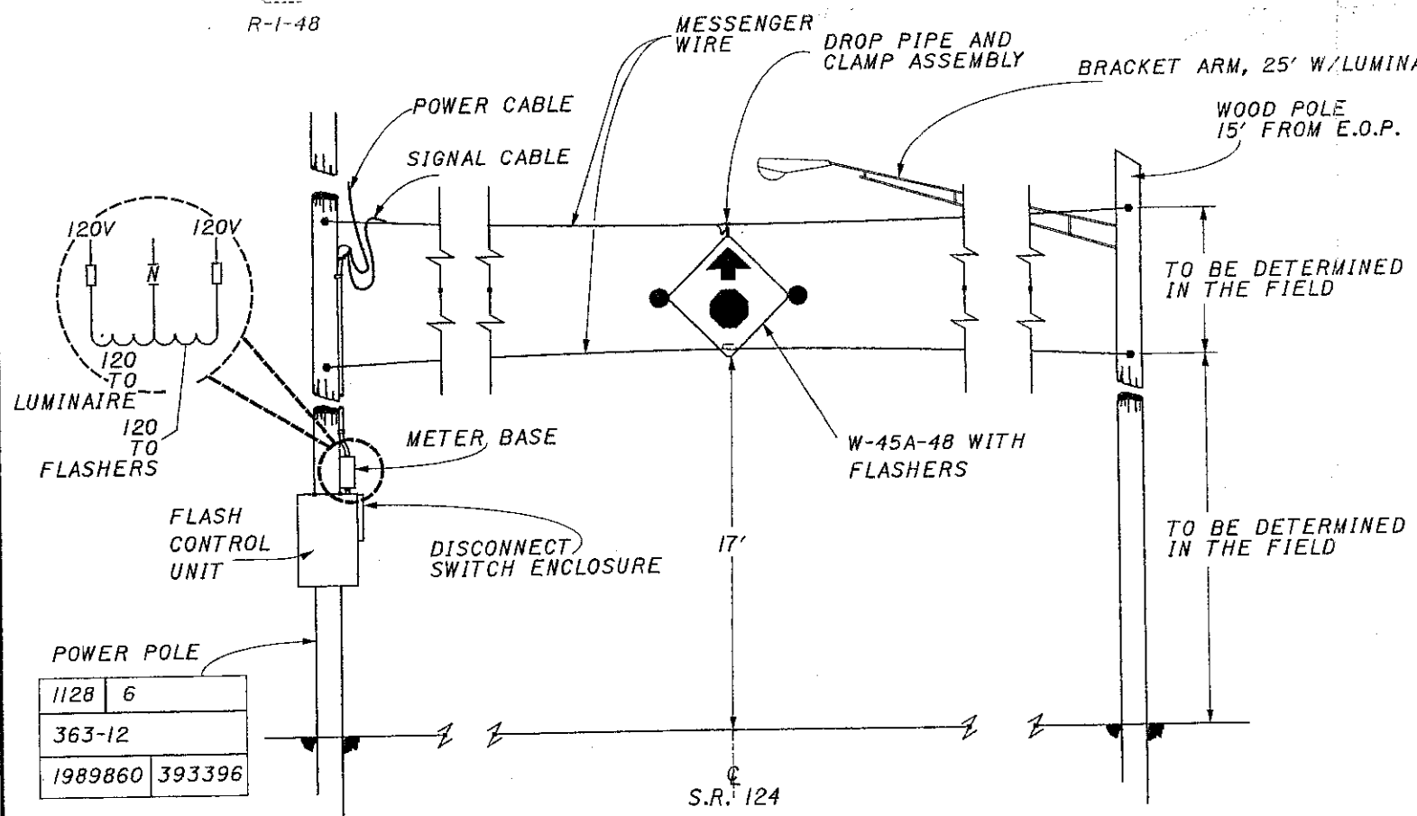
SECTION A-A
