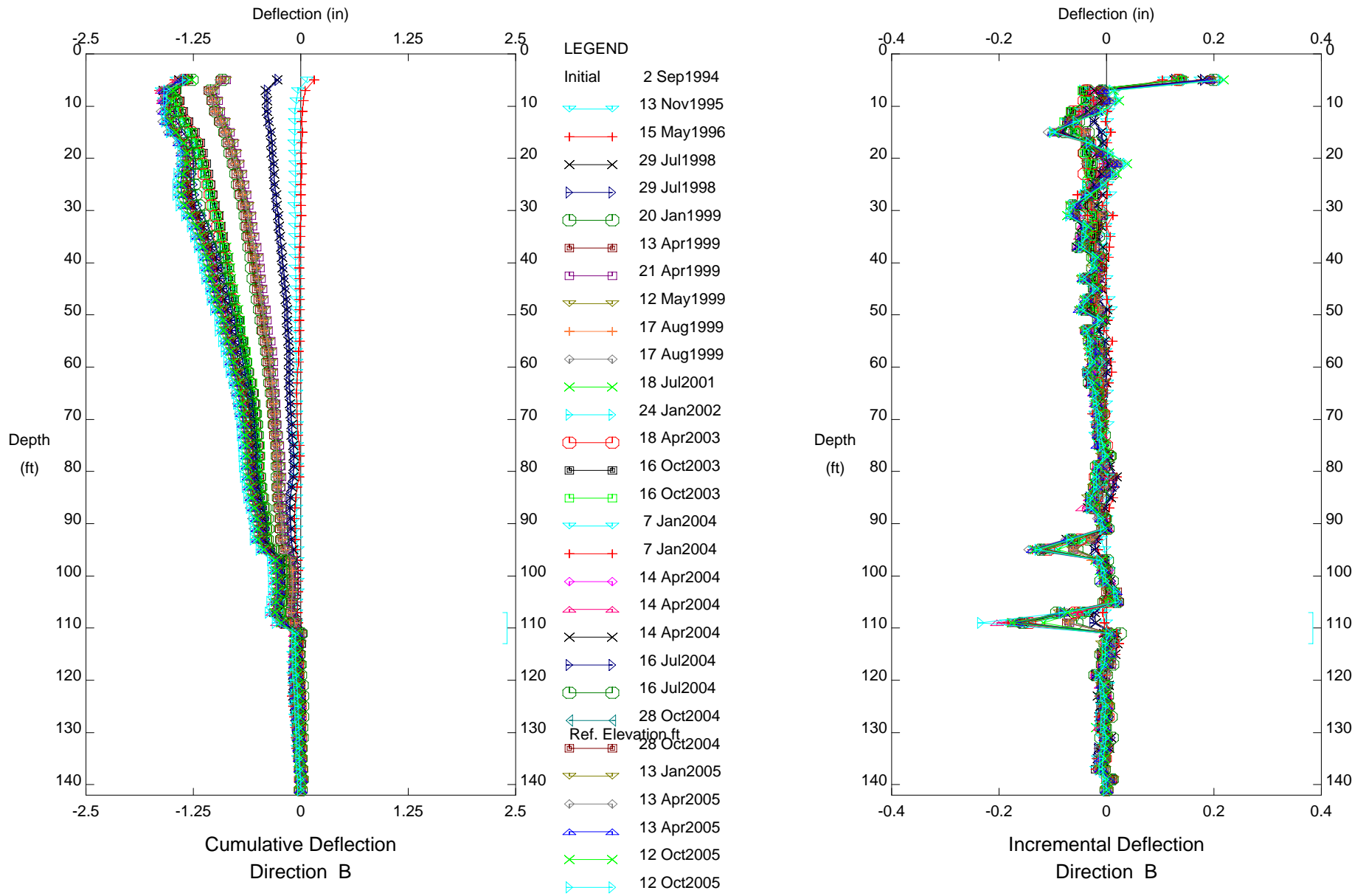
CUY-90, Inclinometer B-105
