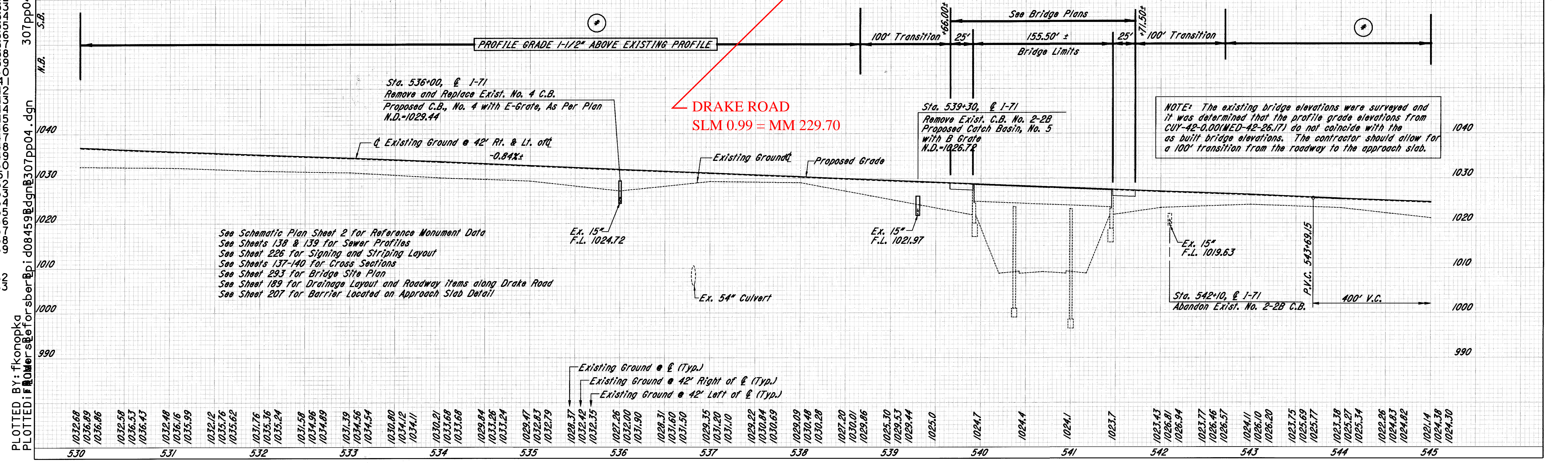
I-71 PLAN & PROFILE STA. 530+00 TO STA. 545+00
