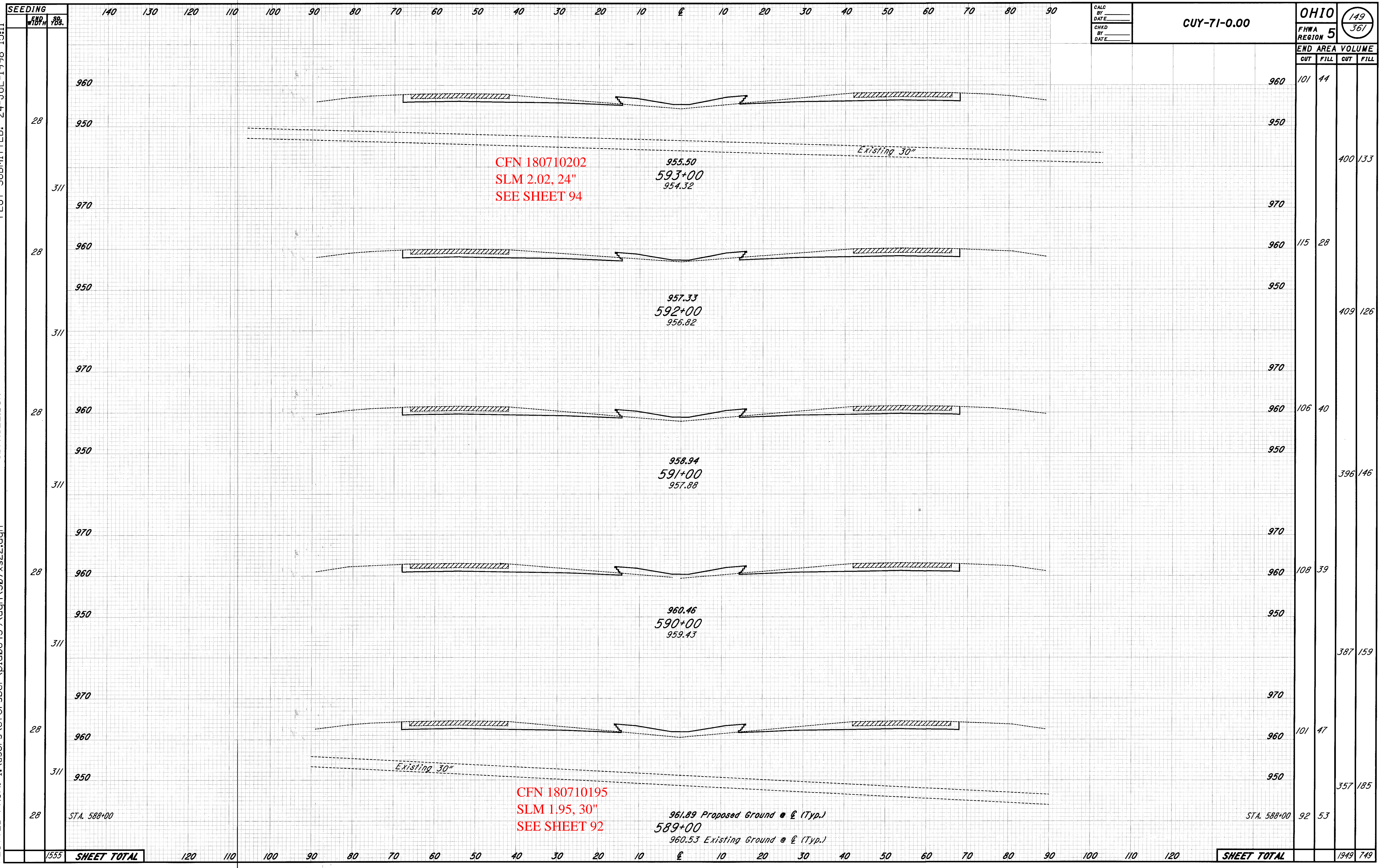
CROSS SECTIONS STA. 589+00 TO STA. 593+00
