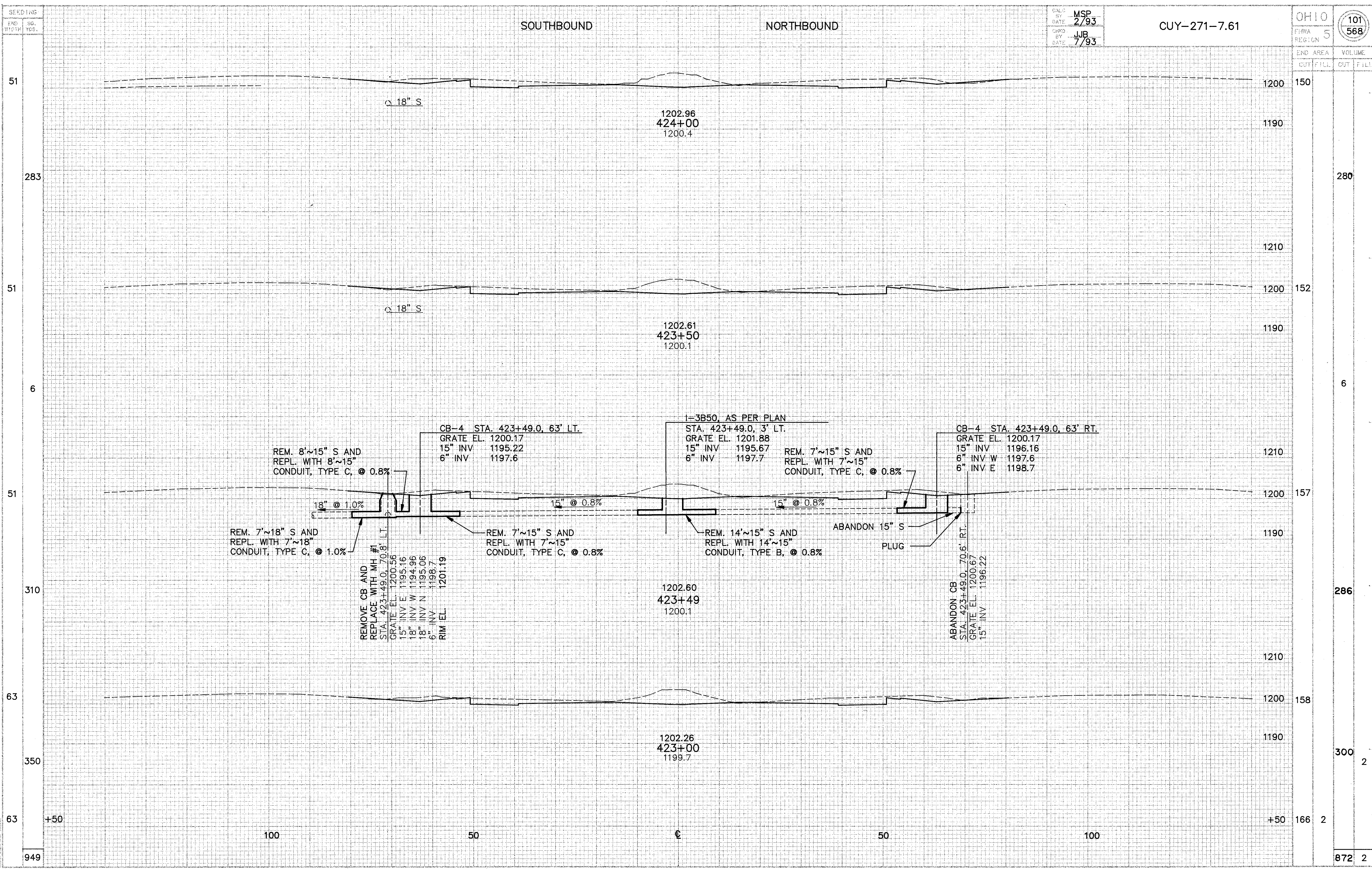
CROSS SECTIONS STA. 423+00 TO STA. 424+00
