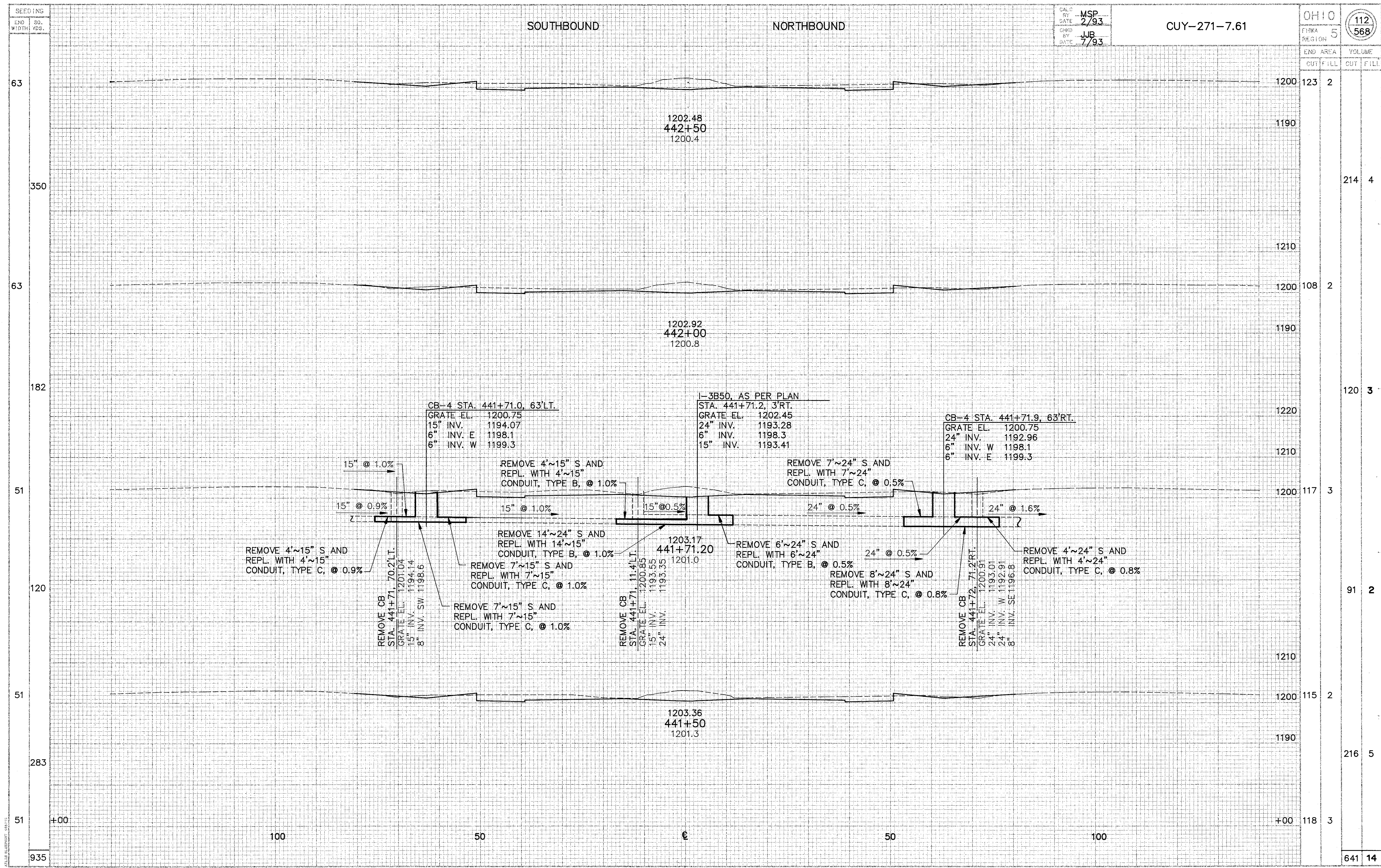
CROSS SECTIONS STA. 441+50 442+50
