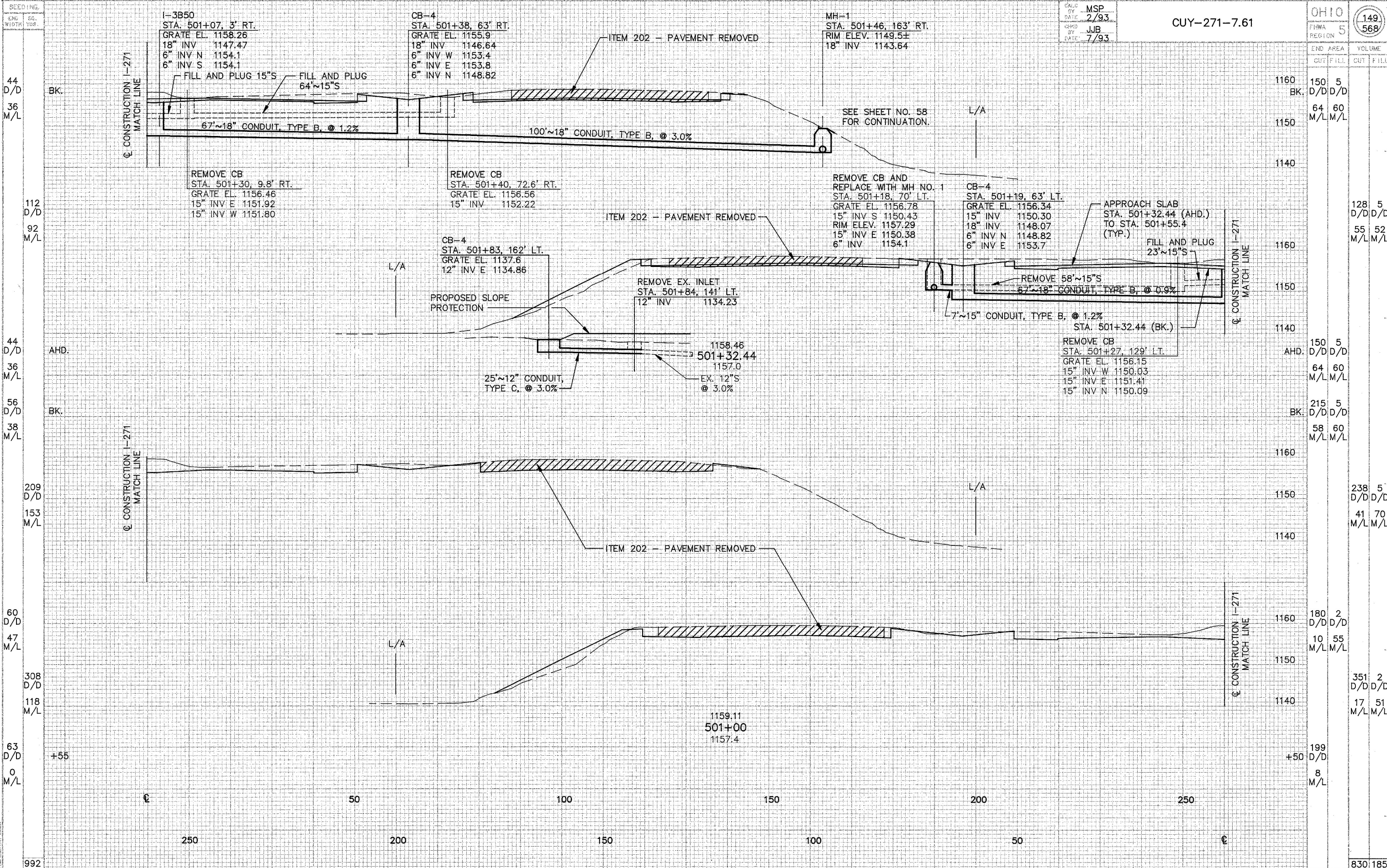
CROSS SECTIONS STA. 501+00 TO STA. 501+32.44
