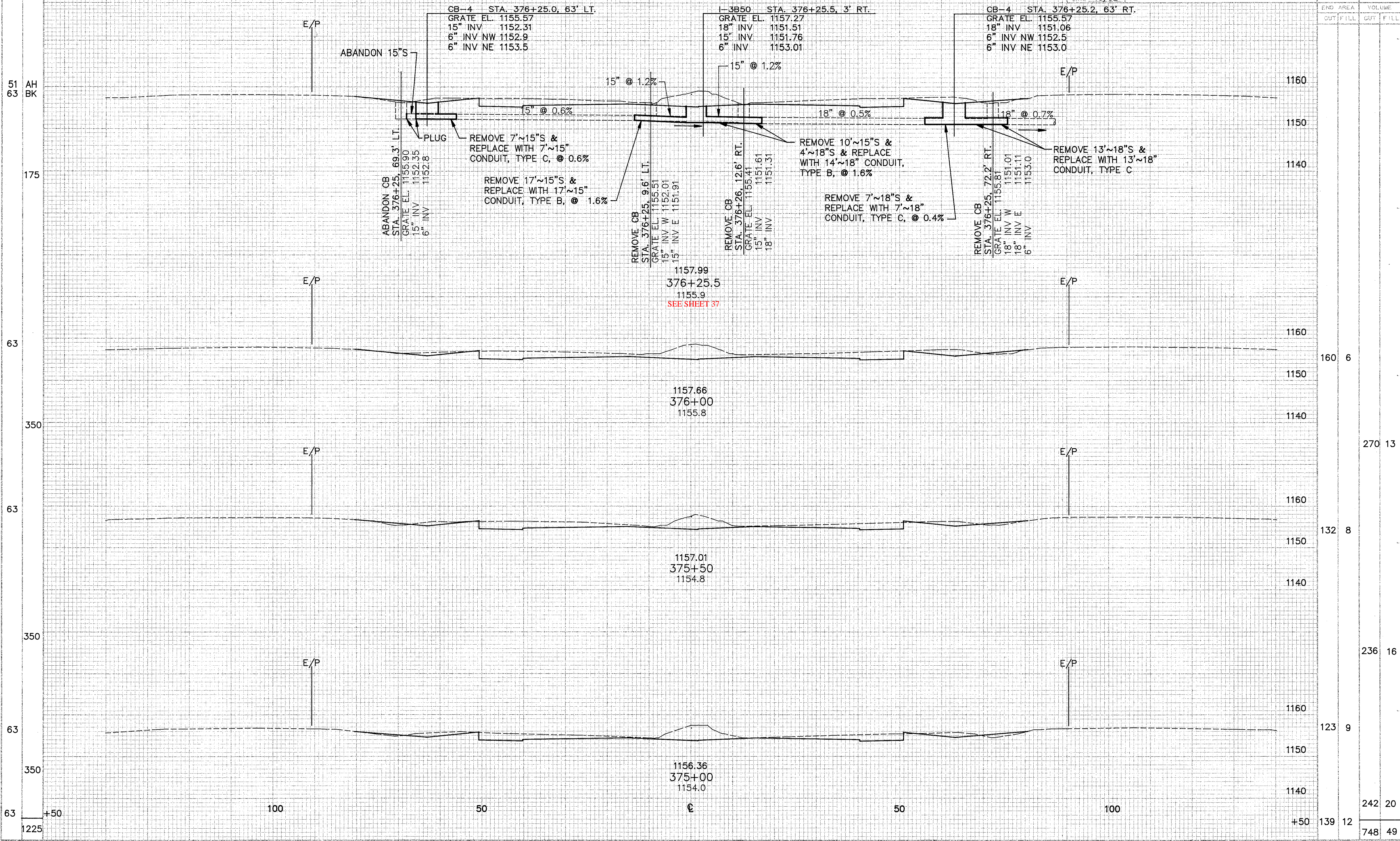
CROSS SECTIONS STA. 375+00 TO STA. 376+25.5
