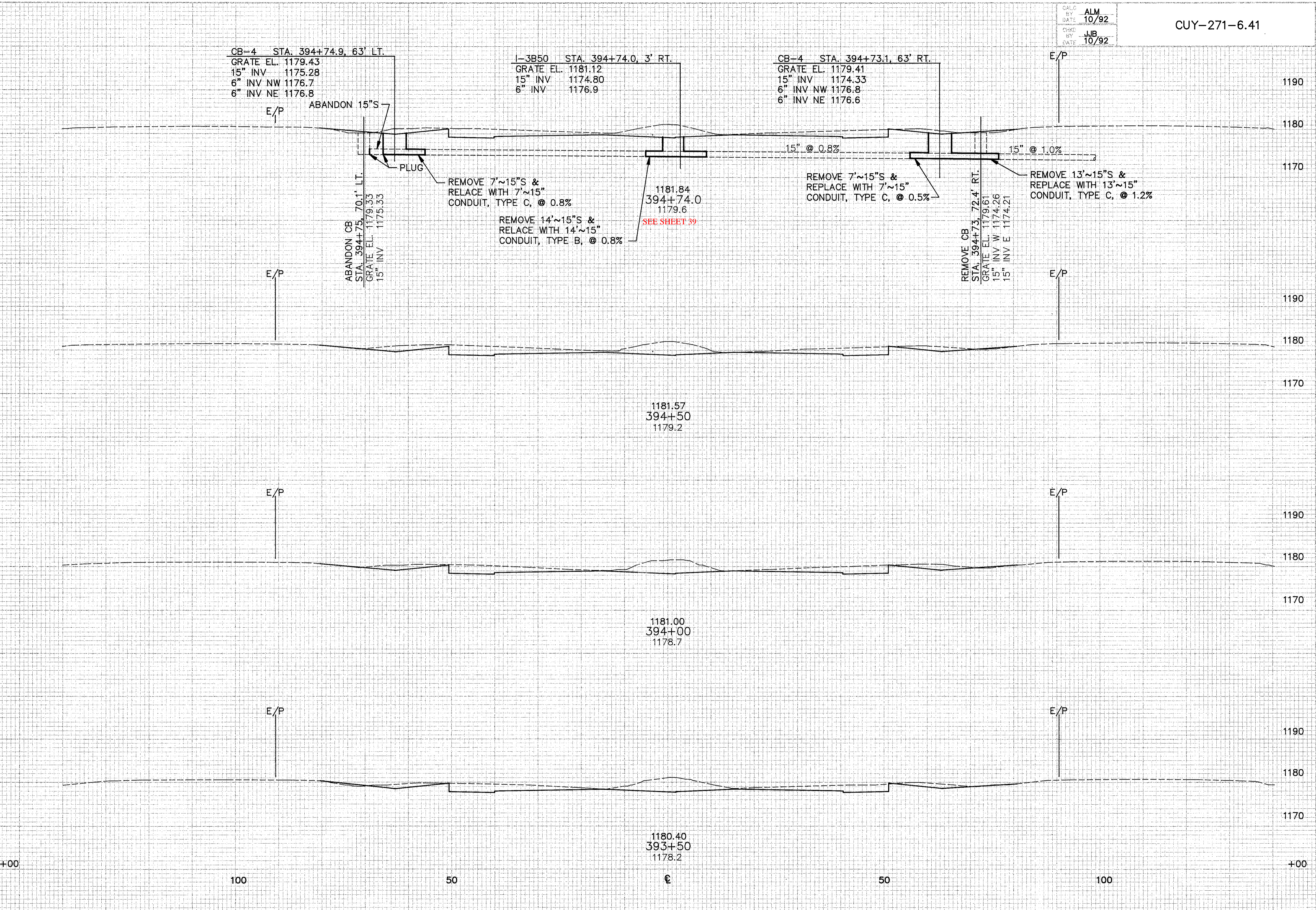
CROSS SECTIONS STA. 393+50 TO STA. 394+74
