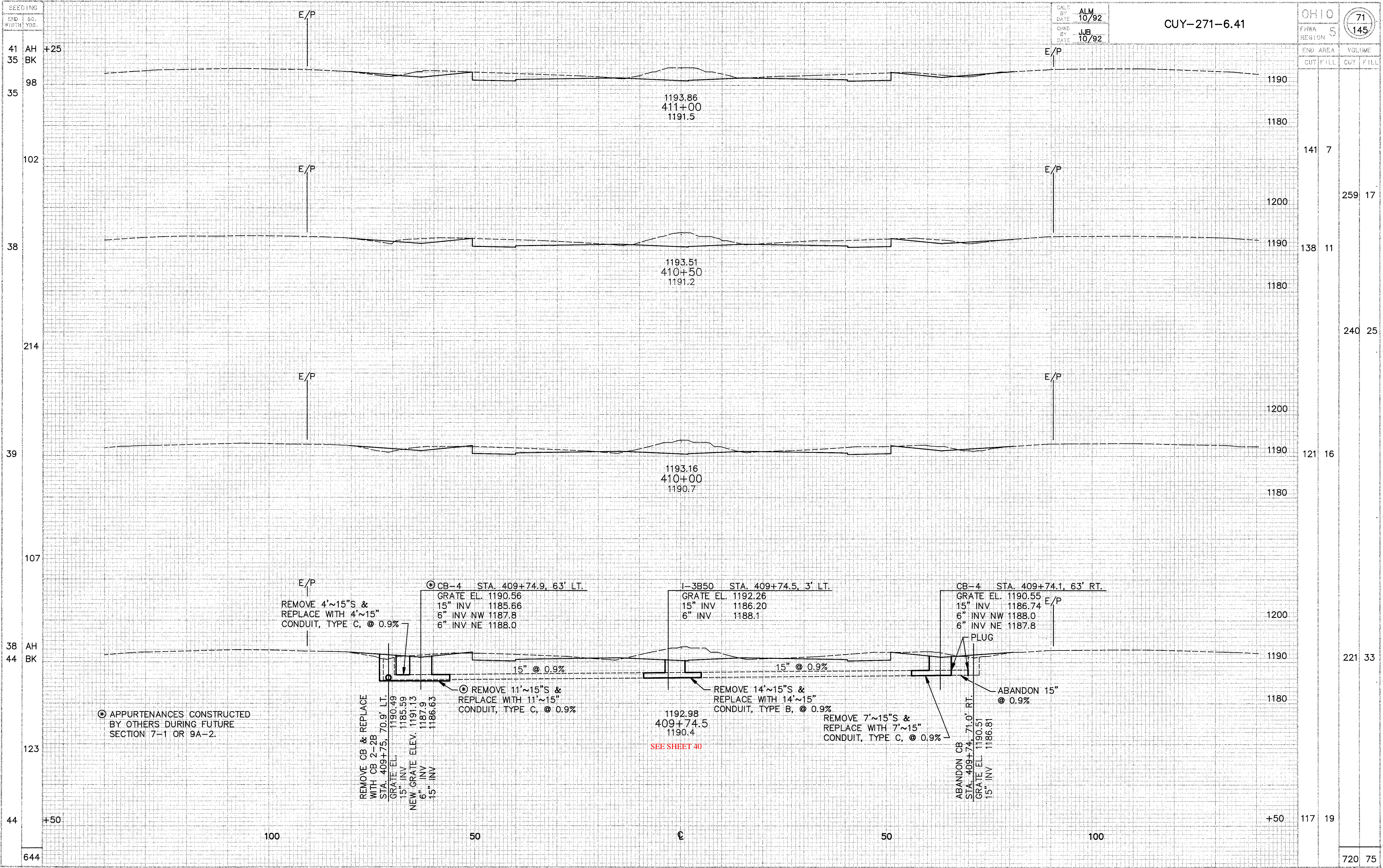
CROSS SECTIONS STA. 409+74.50 TO STA. 411+00
