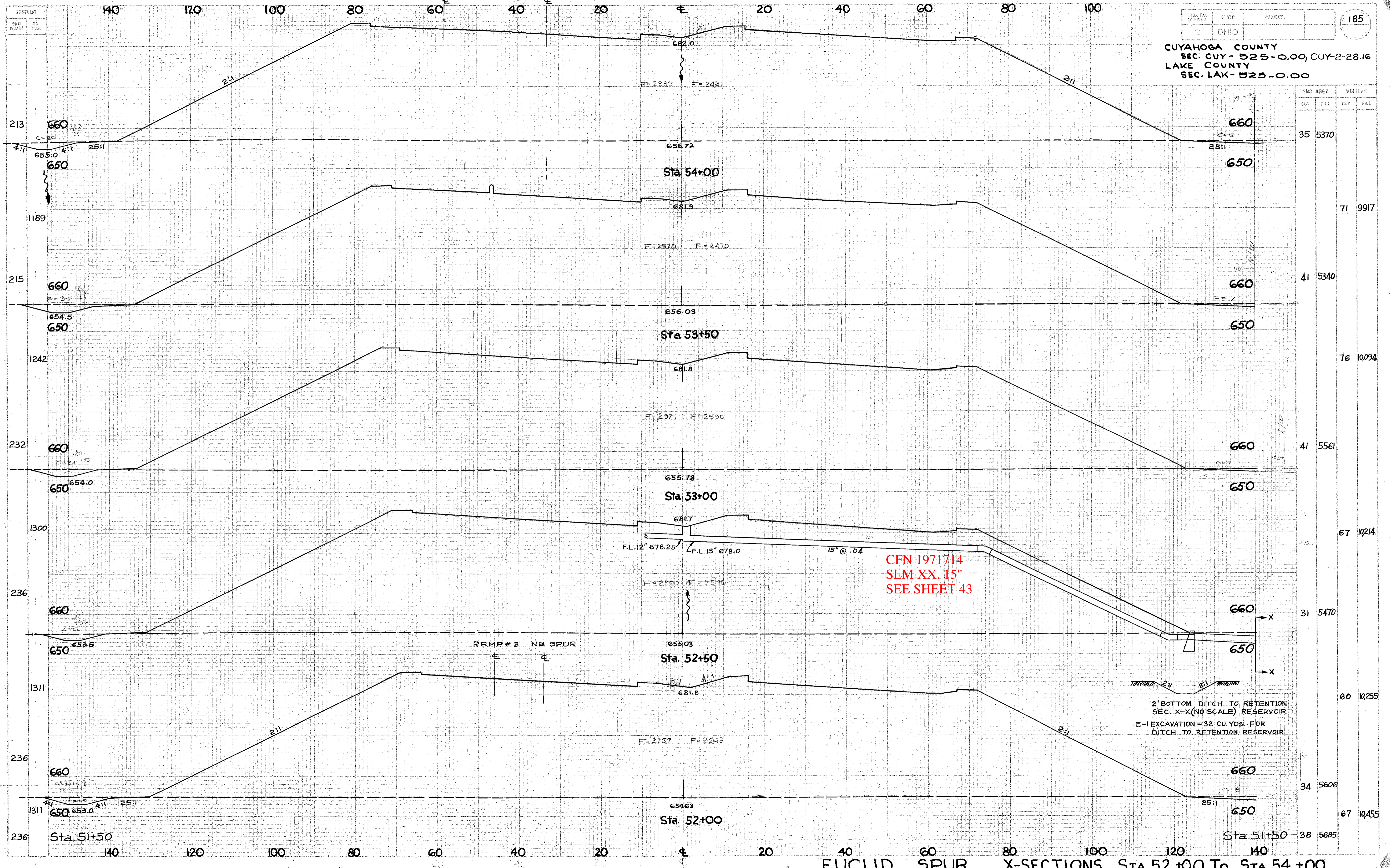
EUCLID SPUR X-SECTIONS STA. 52+00 TO STA. 54+00
