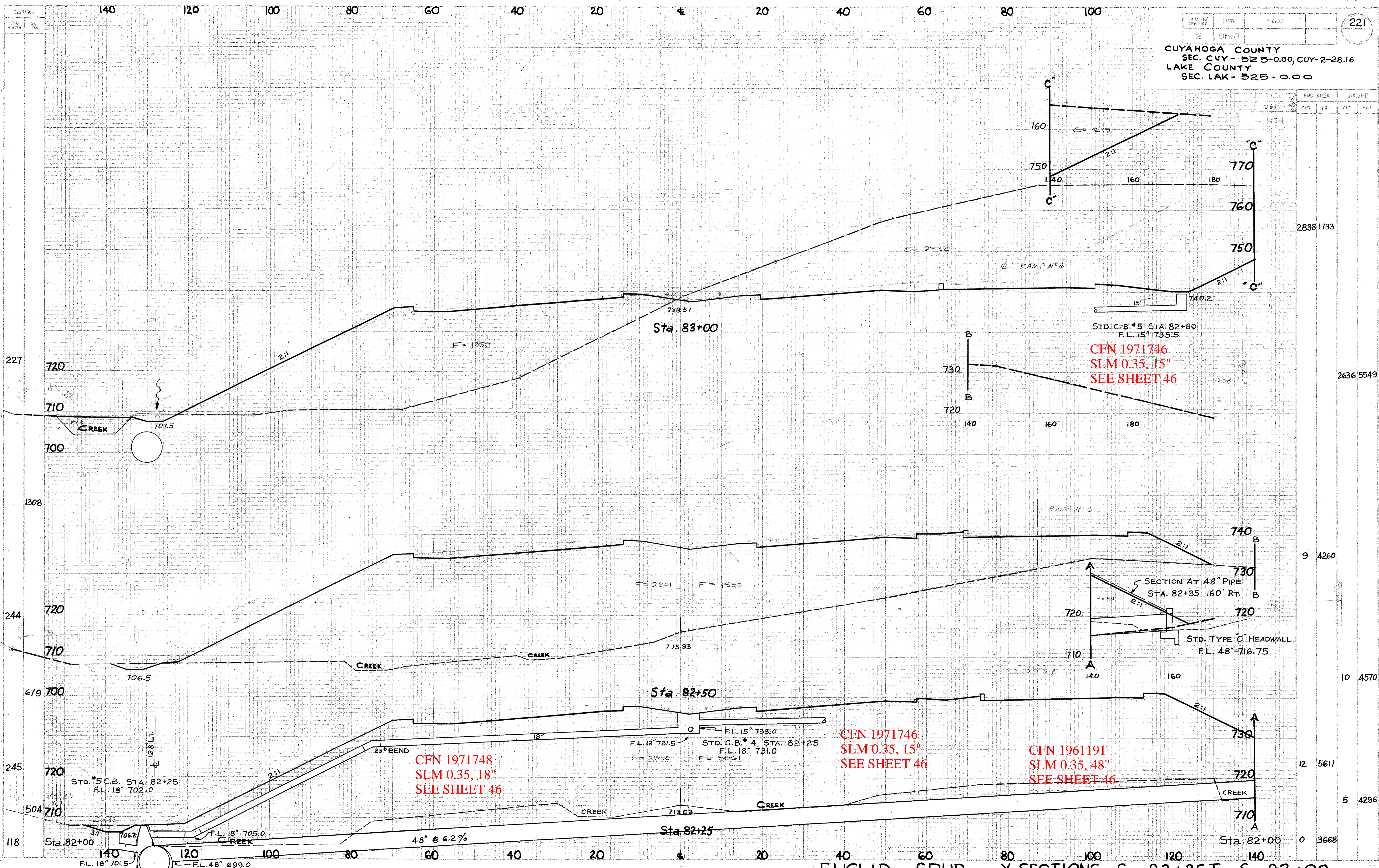
EUCLID SPUR X-SECTIONS STA. 82+25 TO STA. 83+00
