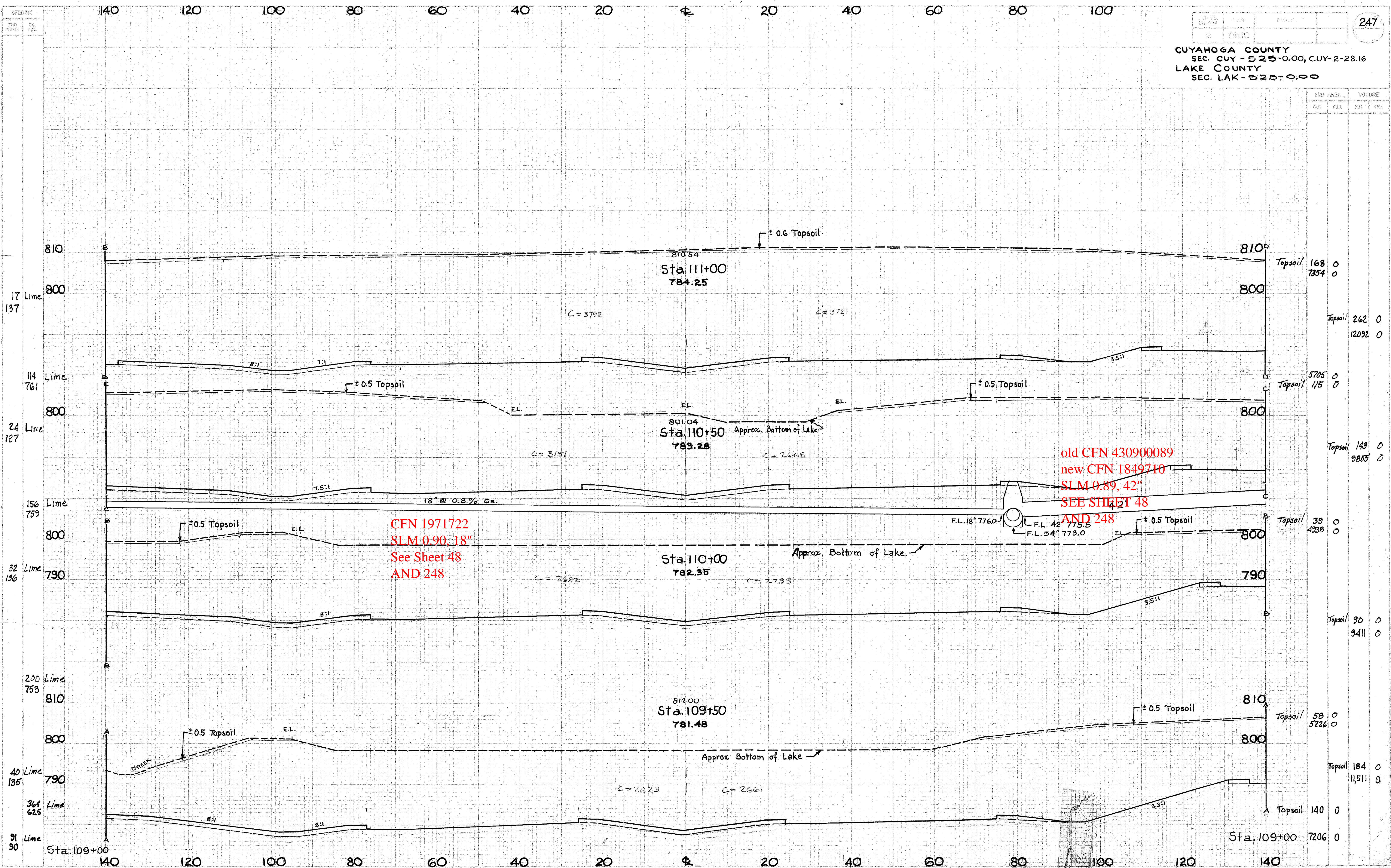
EUCLID SPUR X-SECTIONS STA. 109+50 TO STA. 111+00
