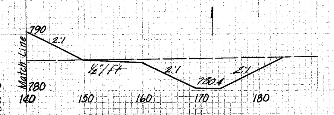
CROSS-SECTIONS STA. 538+00 TO STA. 539+00
