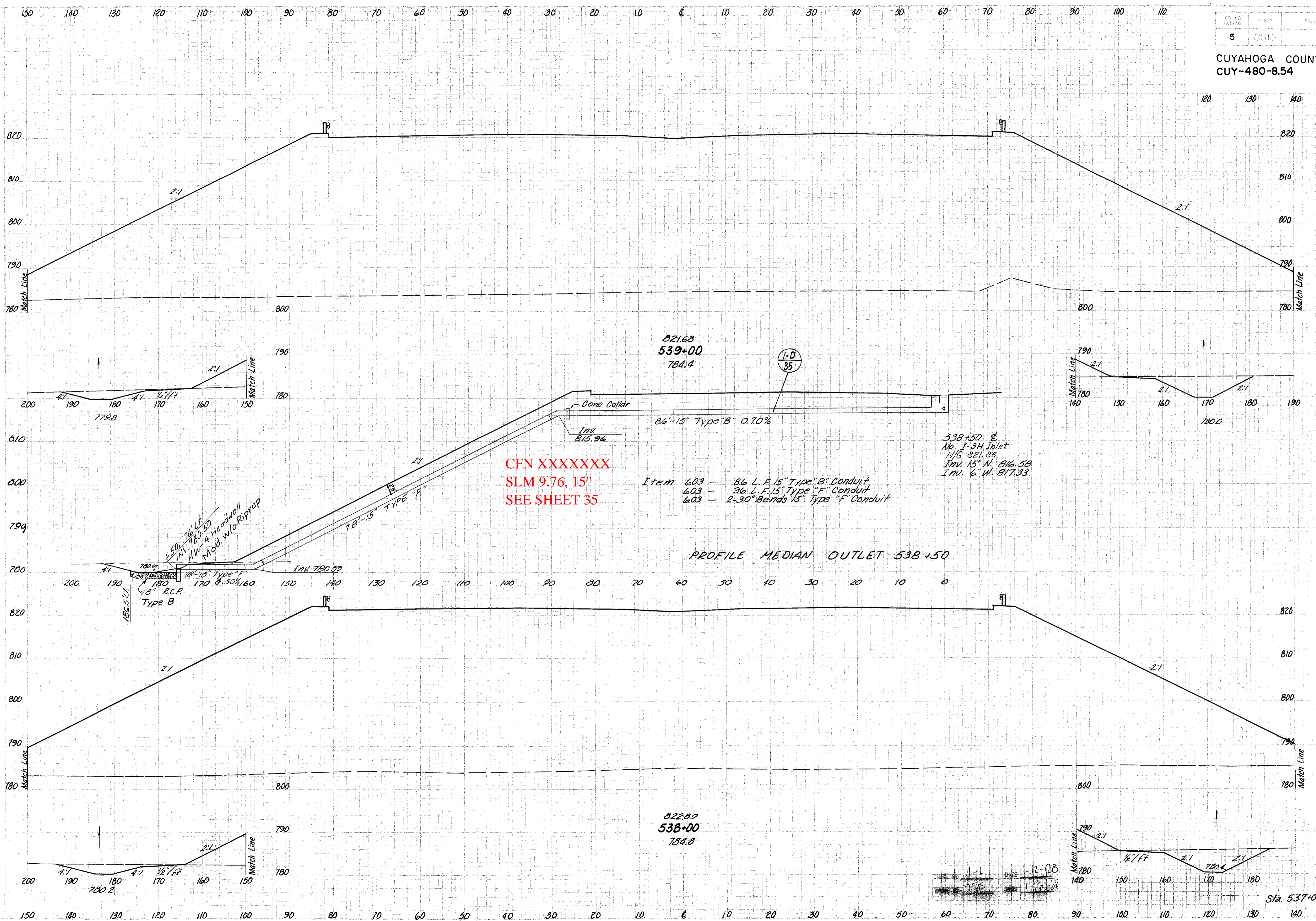
CROSS-SECTIONS STA. 538+00 TO STA. 539+00
