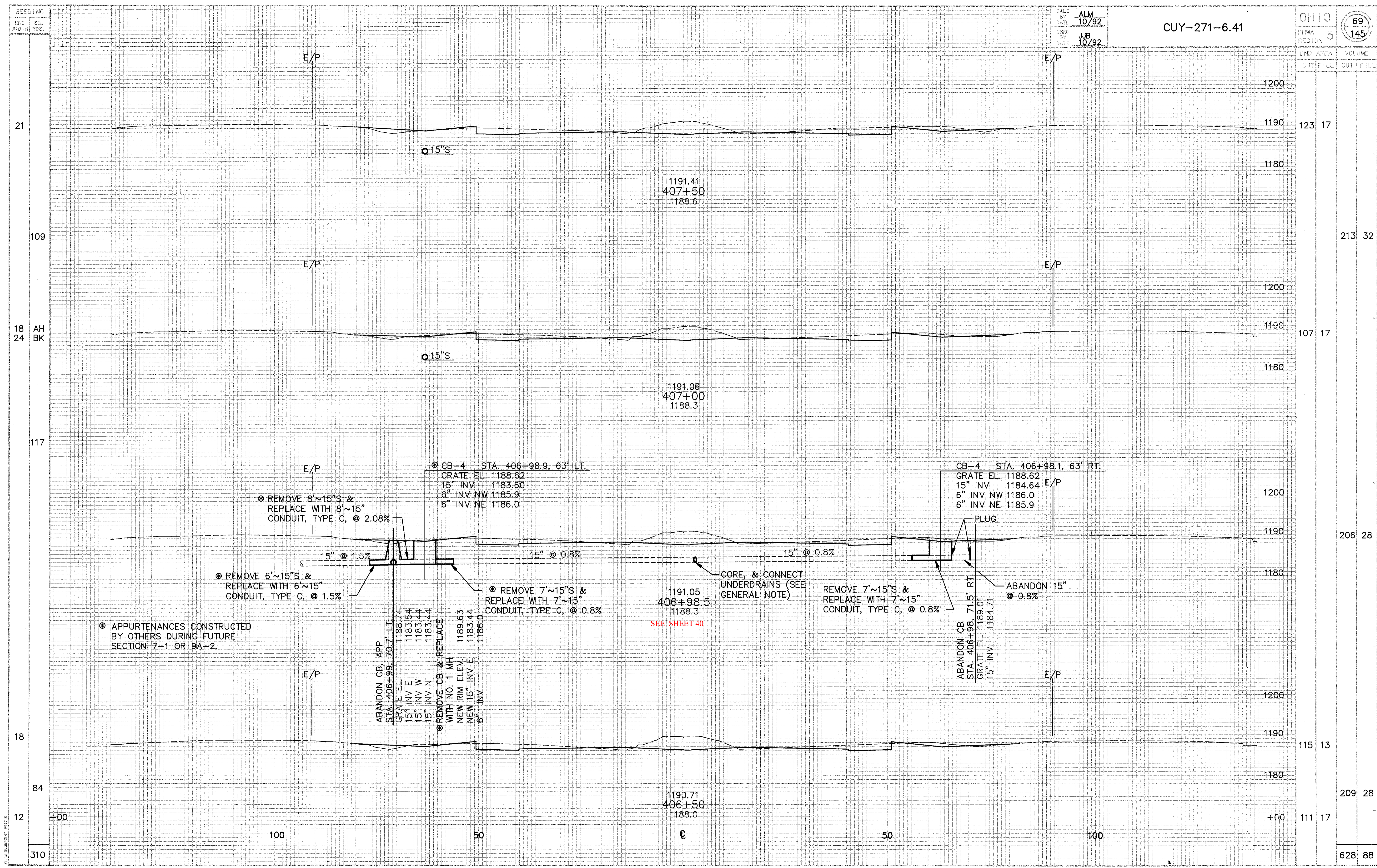
CROSS SECTIONS STA. 406+50 TO STA. 407+50
