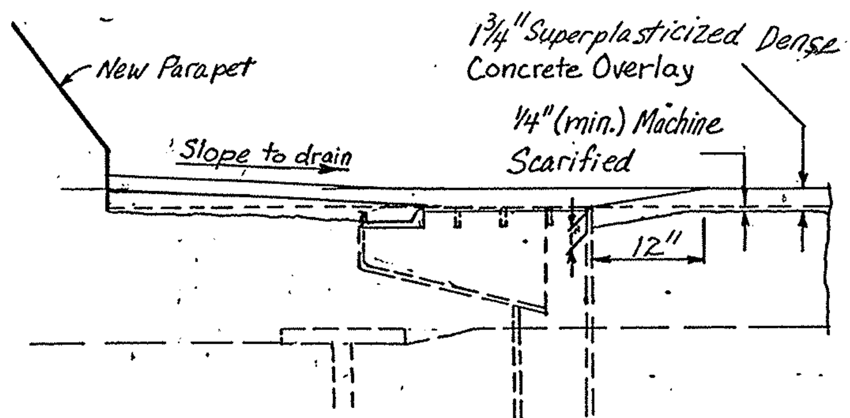
SECTION A-A
