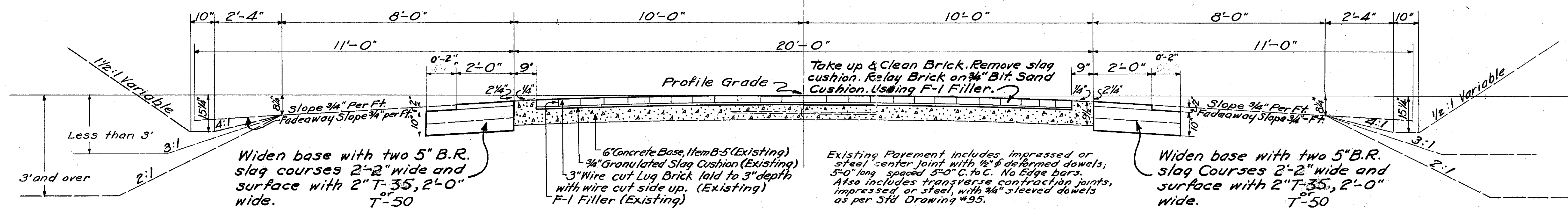
Sec. F2 (Pt.) Sta. 0+00 to Sta. 18+50
