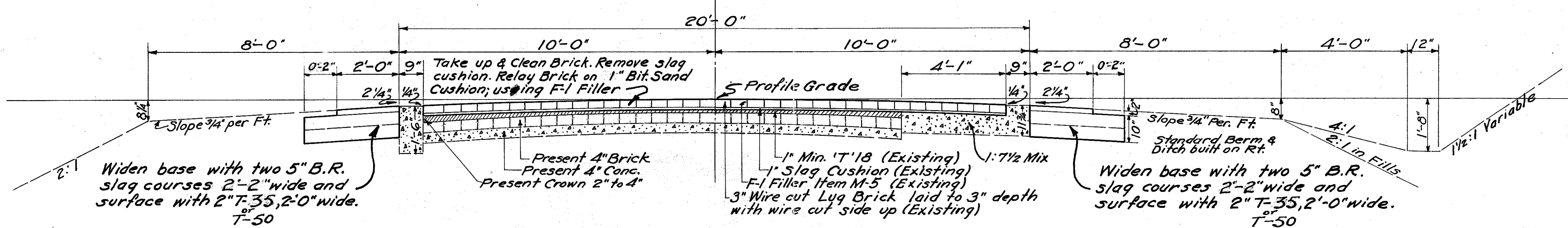
Sec. F-1 (Pt.) Parral, F-2 (Pt.) Sta. 25+00 to Sta. 101+78.45
