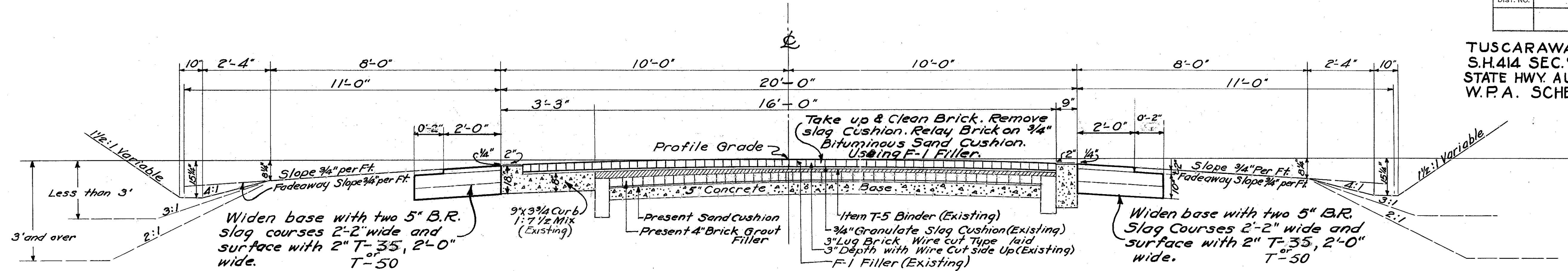
Sec. F2 (Pt.) Sta. 18+50 to Sta. 46+00
